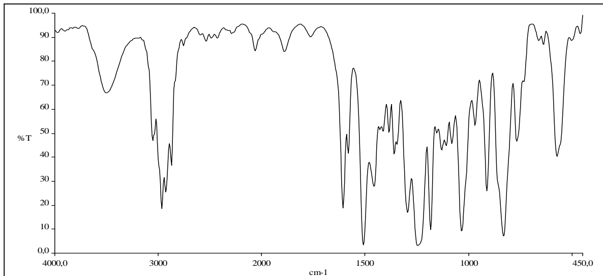
Espectro de infravermelho da resina epóxi (comp. B).
