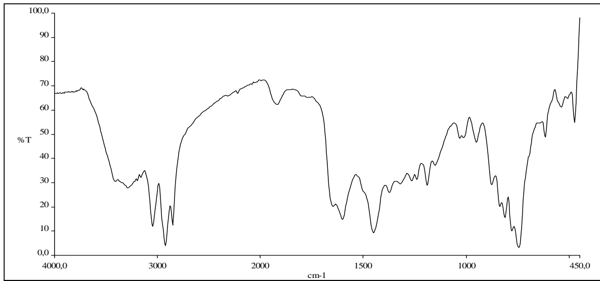
Espectro de infravermelho da mistura das resinas de poliamida e alcatrão de hulha (comp. A).
