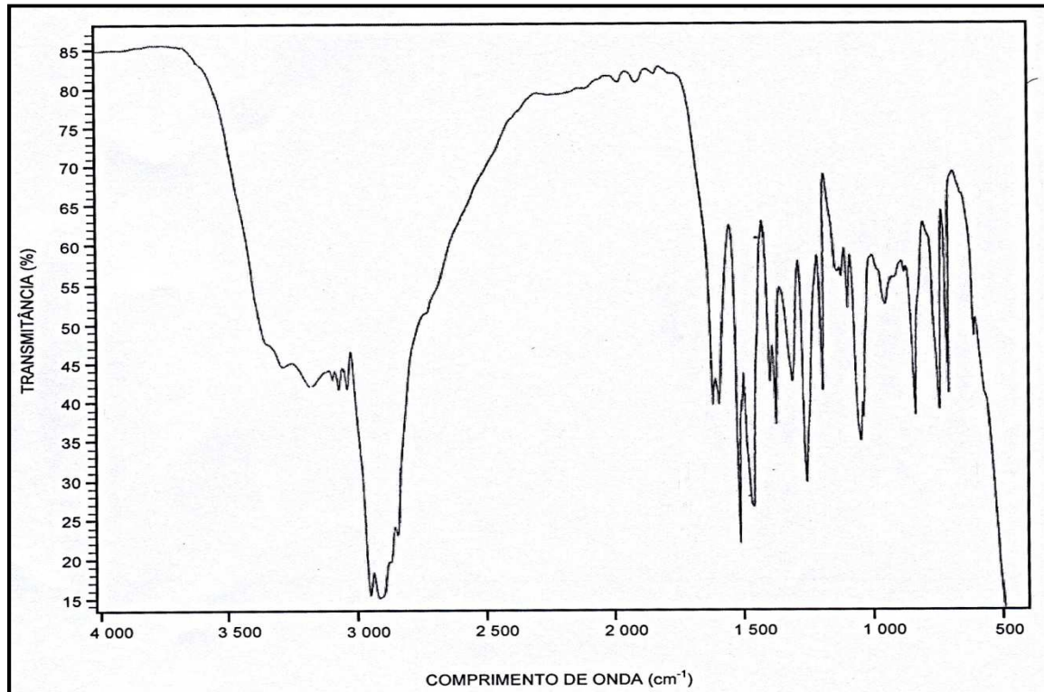
Espectro de infravermelho da resina poliamina (comp. B) - Gráfico 1.
