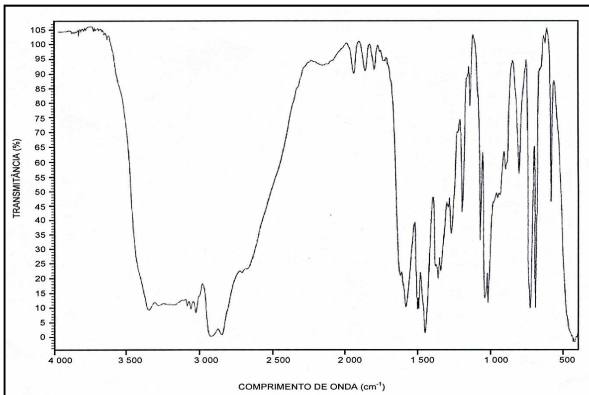
Espectro de infravermelho da resina poliamina (comp. B) - Gráfico 2.
