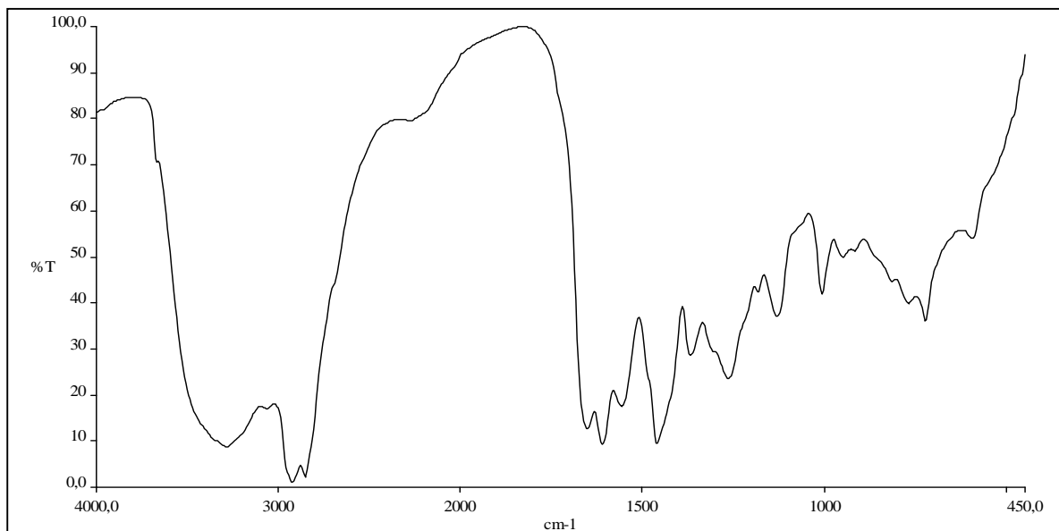
Espectro de infravermelho de resina poliamida (comp. B) – Gráfico 2.
