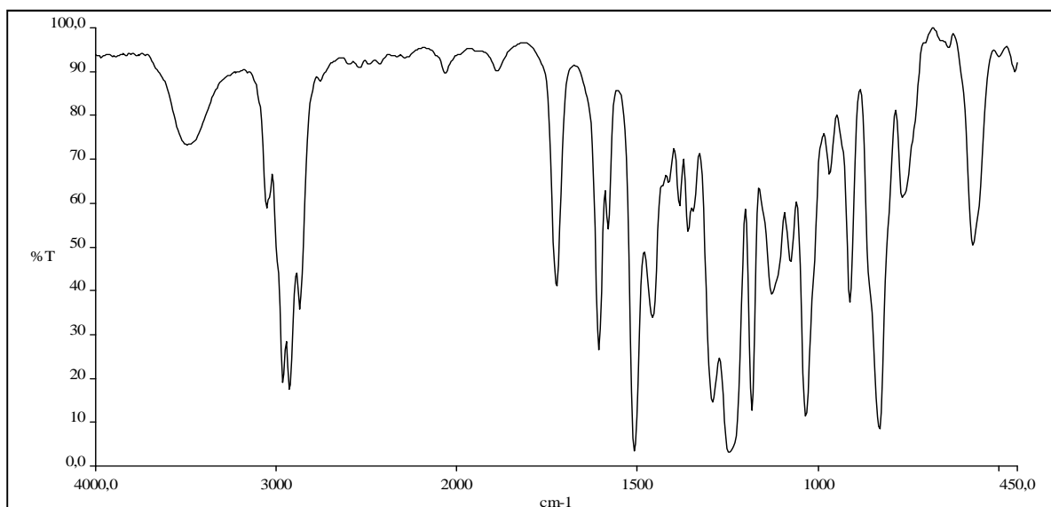
Espectro de infravermelho da resina epóxi (comp. A) – Gráfico 2.
